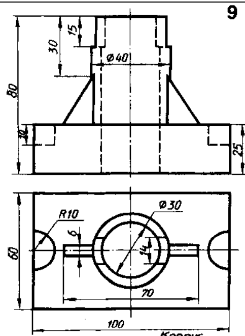
Корпус
