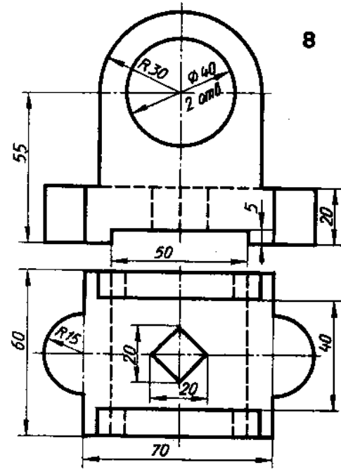
Опора
