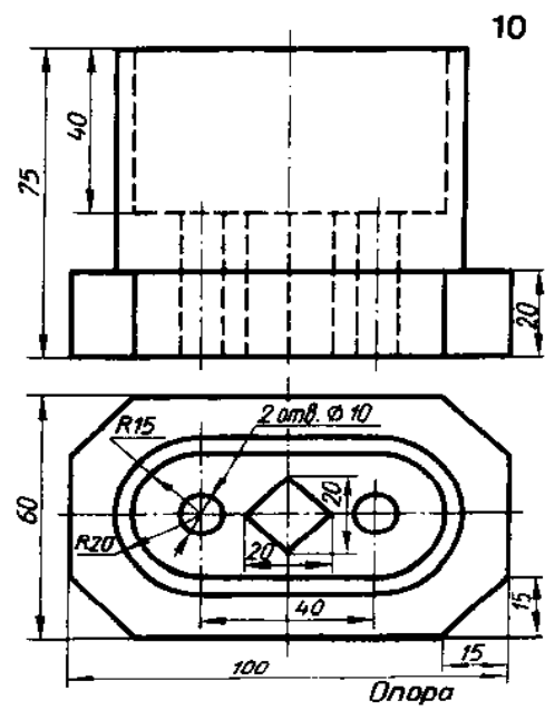
Опора
