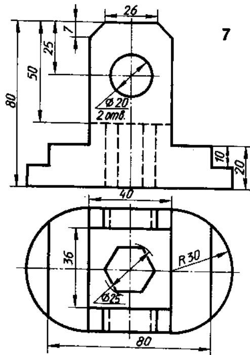
Подставка
